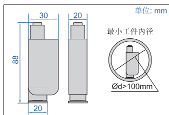
主机尺寸图
